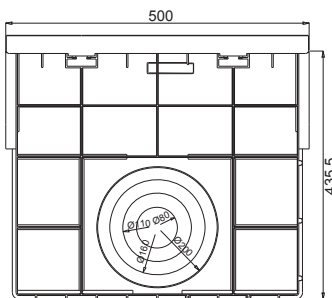
vooraanzicht
