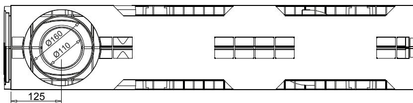
onderaanzicht
