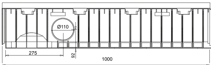
zij-aanzicht
