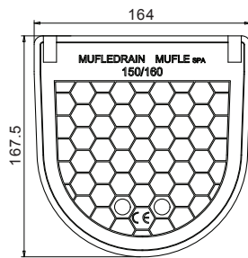
eindkap
