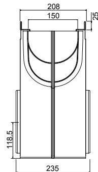
zij-aanzicht
